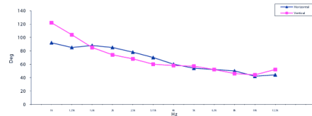
ШИРИНА ПУЧКА
