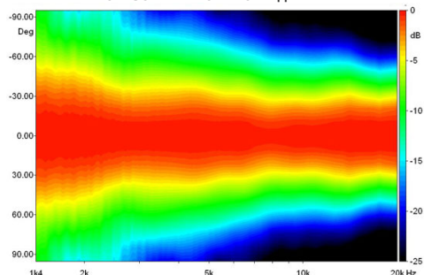
ГОРИЗОНТАЛЬНОЕ РАСПРЕДЕЛЕНИЕ
