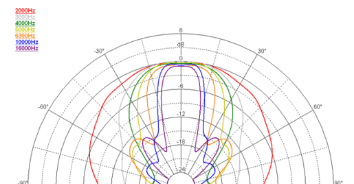
DIAGRAMMA POLARE VERTICALE
